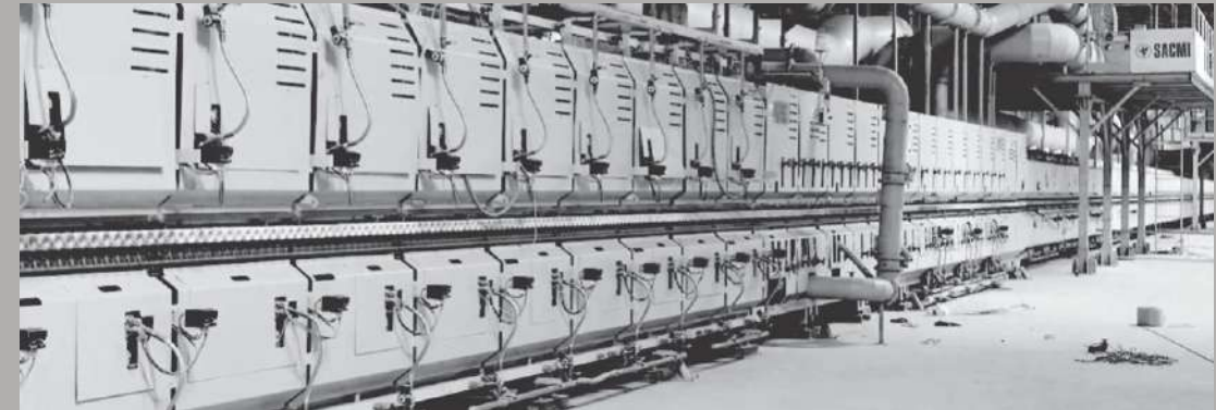
SACMI KILN
